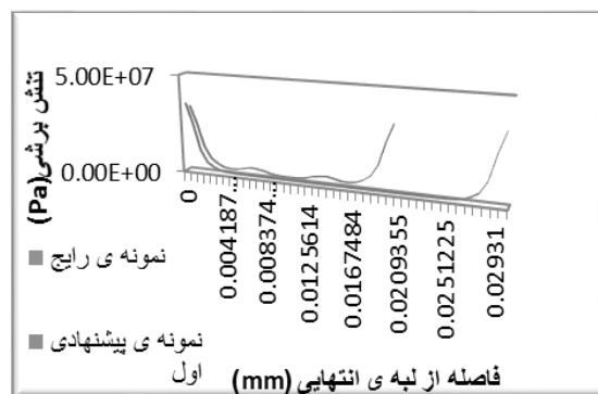
شکل (۸) مقایسه توزیع تنش برشی در حالت رایج و پیشنهادی در طول اتصال یکسان
