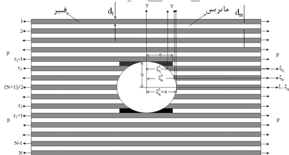
شکل (۶) موقعیت مختصات محلی هر فیبر در تک لایه مرکب با الیاف پیوسته.
