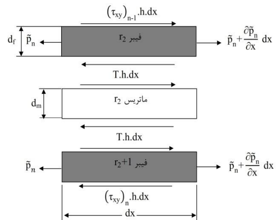
شکل (۴) المانی از فیبرهای نوع (ج) و نیروهای وارد بر آنها (فیبر r_2 ).
