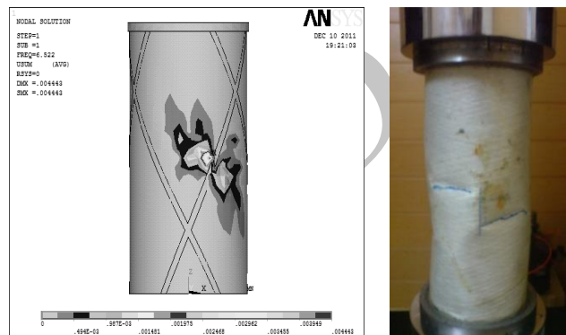
شکل (۶): نمونه ساخته شده تحت بار محوری به همراه مدل اجزاء محدود آن.
