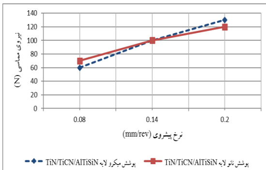
شکل (۶) تأثیر نرخ پیشروی بر نیروی محوری ابزار در شرایط ماشینکاری با عمق برشی ۰/۵ میلی متر و سرعت برشی ۵۰ متر بر دقیقه.
