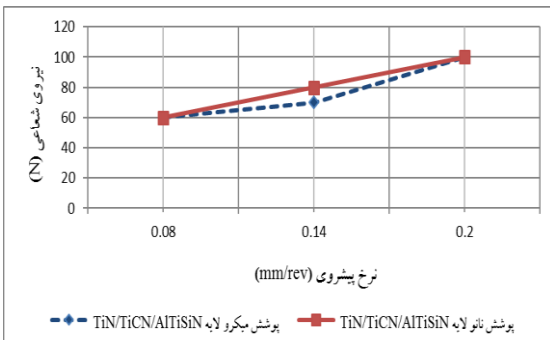
شکل (۵) تأثیر نرخ پیشروی بر نیروی محوری ابزار در شرایط ماشینکاری با عمق برشی ۰/۵ میلی متر و سرعت برشی ۵۰ متر بر دقیقه.
