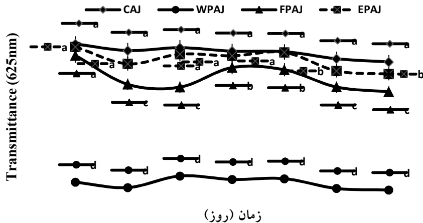
نمودار ۲- تاثیر نوع تیمار در شفافیت آب سیب در طول نگهداری در دمای 25 \pm 5^\circ \text{C}
