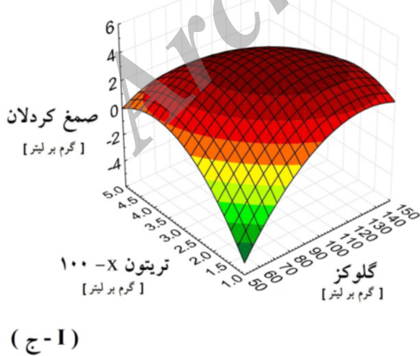
شکل ۷- تاثیر تعاملی متغیرهای موثر گلوکز، عصاره مخمر و تریتون X-100 با استفاده از نمودارهای سطح پاسخ سه بعدی (I) - کنتور (II)
