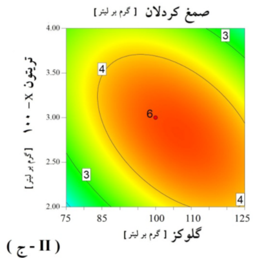
شکل ۷- تاثیر تعاملی متغیرهای موثر گلوکز، عصاره مخمر و تریتون X-100 با استفاده از نمودارهای سطح پاسخ سه بعدی (I) - کنتور (II)
