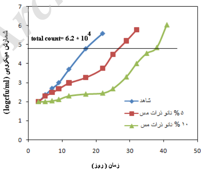
شکل ۳- نتایج شمارش باکتری شیر بسته بندی شده در پلاستیک‌های نوع معمولی و حاوی نانو ذرات مس (۵ و ۱۰٪ وزنی)
