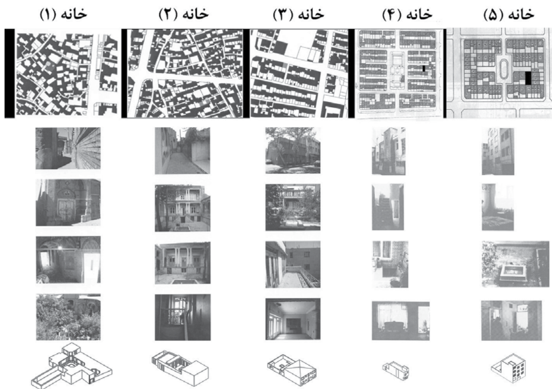
عکس ۱۱. نقشه موقعیت خانه‌های شماره ۱ الی ۵ در بافت شهری به همراه ایزومتریک؛ مأخذ عکس‌ها: خانه‌های شماره ۱ الی ۳: شلویری، یوهانس. خانه‌های شماره ۴ و ۵: دشتی)؛ مأخذ: نگارندگان.
