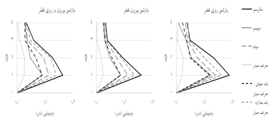
شکل ۱۰. میزان تغییر مکان ماکزیمم طبقات مختلف قاب با سیستم دیوار برشی فولادی با سه چیدمان مختلف بازشوهایی چندگانه
