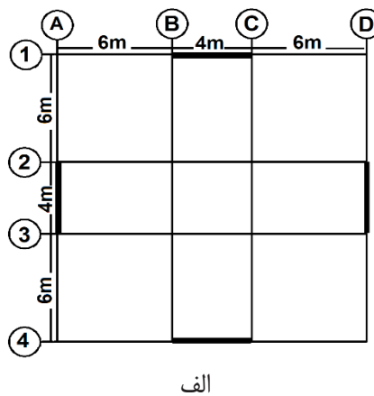
شکل ۱. الف) پلان طبقات ساختمان
