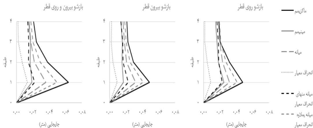
شکل ۹. میزان پراکندگی پاسخ طبقات مختلف قاب با سیستم دیوار برشی فولادی با سه چیدمان مختلف بازشوهای چندگانه
