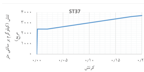
شکل ۷. منحنی رفتاری فولاد مورد استفاده
