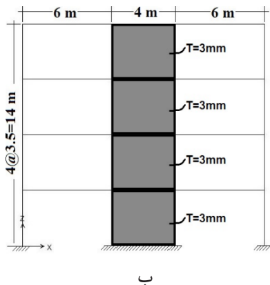
ب) نمای قاب برگرفته از ساختمان ۴ طبقه
