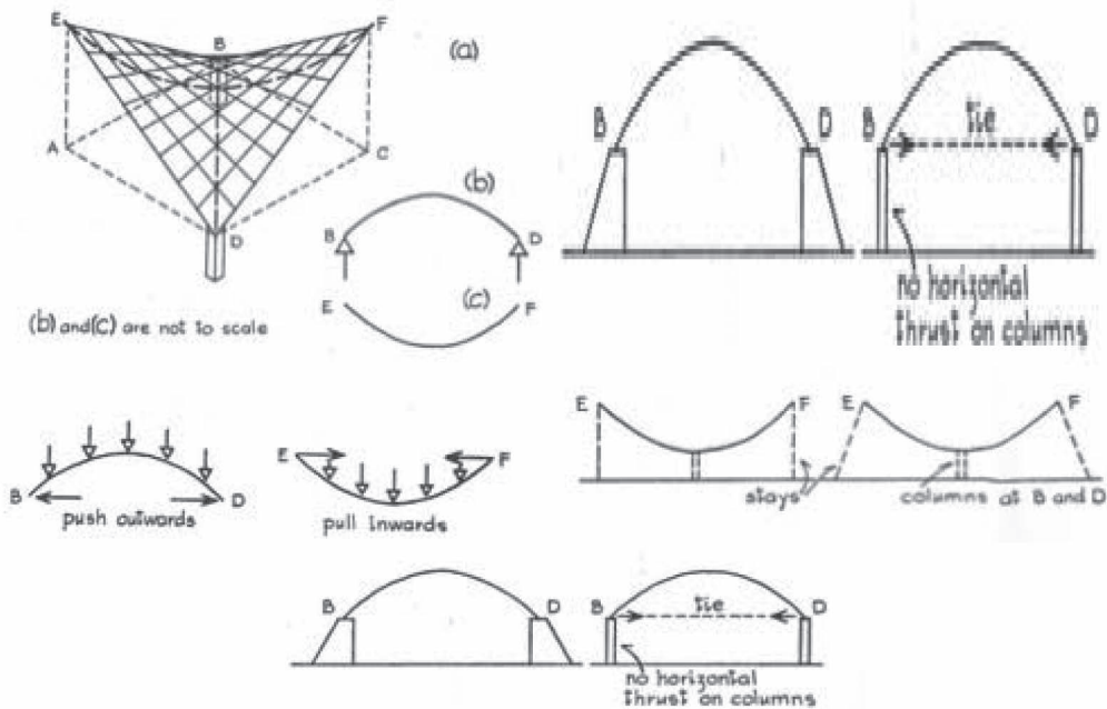
تصویر ۴ الی ۸. تحلیل سازه‌ای معماری سقفهای پوسته‌ای؛ ماخذ: نگارنده.
