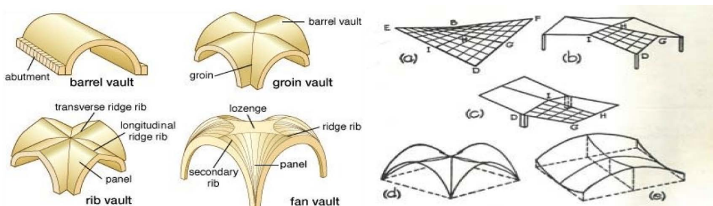
تصویر ۴ الی ۸. تحلیل سازه‌ای معماری سقفهای پوسته‌ای؛ ماخذ: نگارنده.
