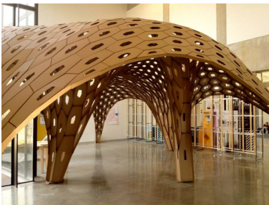
تصویر ۲۱. نمونه‌هایی از سقف پوسته‌ای چوبی؛ ماخذ: نگارنده.
