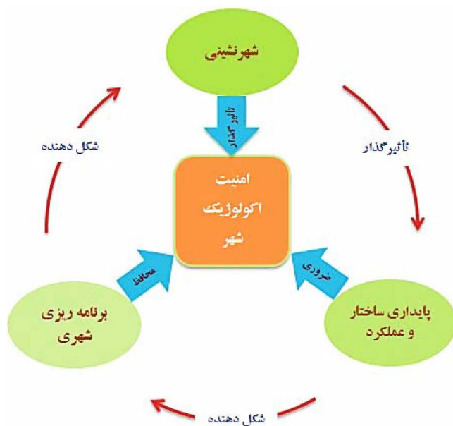
نمودار ۲. رابطه بین شهرنشینی، برنامه‌ریزی شهری و پایداری ساختار و عملکرد با امنیت اکولوژیک شهر؛ مأخذ: Linyu & Zhaoxue, 2010:1394
