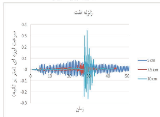
شکل ۲۳. سرعت در مقابل زمان برای سازه های پوسته ای
