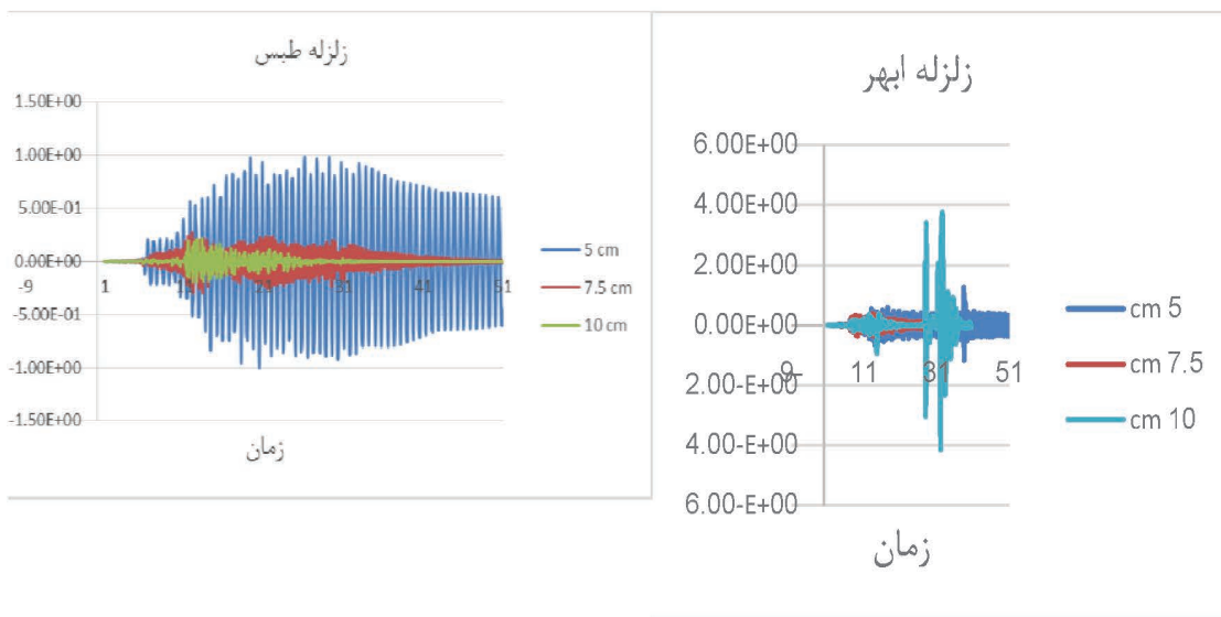
شکل ۱۶. شتاب در مقابل زمان برای سازه های پوسته ای تحت رکورد زلزله طبس
