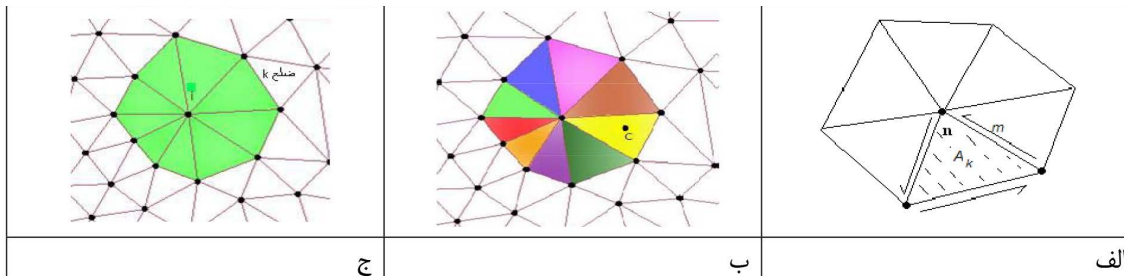
شکل ۳. حجم کنترل های مورد استفاده در شبکه مثلثی بیساختار الف- المان مثلثی با مساحت مقادیر مشتقات (جابجایی) کرنش) در مراکز المان ب- حجم کنترل فرعی محاسبه Ak ج- حجم کنترل اصلی برای محاسبه مقادیر جابجایی در نقاط گرهی (رتوس المان).
