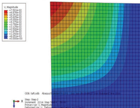
شکل ۲۲. سرعت ایجاد شده در پوسته بتنی با ضخامت ۵ cm
