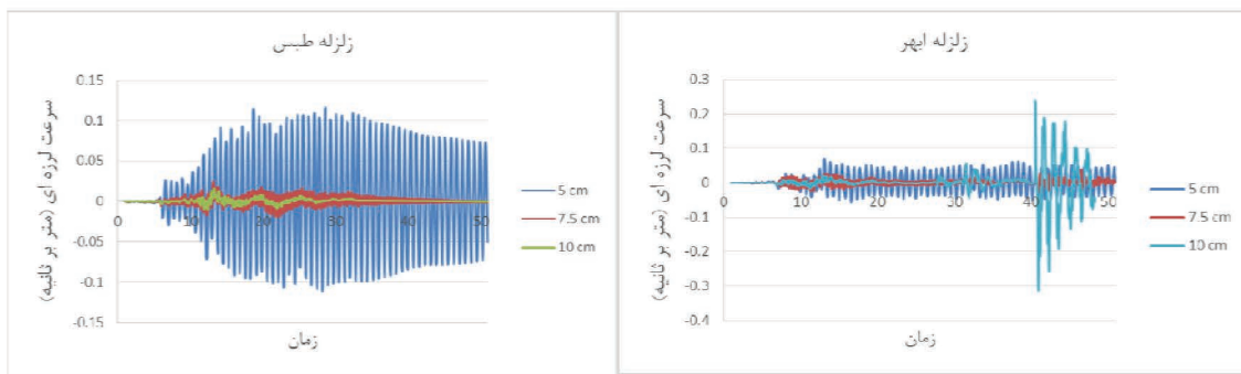
شکل ۲۰. سرعت در مقابل زمان برای سازه های پوسته ای
