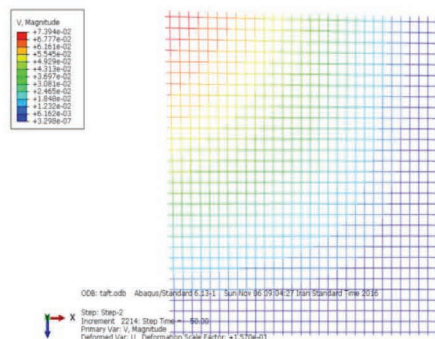
شکل ۲۴. سرعت ایجاد شده در میلگردهای تقویت، پوسته بتنی با ضخامت ۵ cm تحت زلزله تفت
