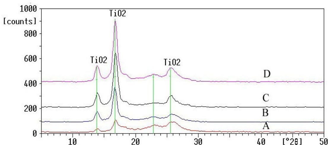
شکل ۳. گراف XRD منسوج PLA لایه نشانی شده با TiO_2 در زمانهای ۳ و ۵ و ۱۰ دقیقه به ترتیب (B,C,D) و نمونه خام (A)
