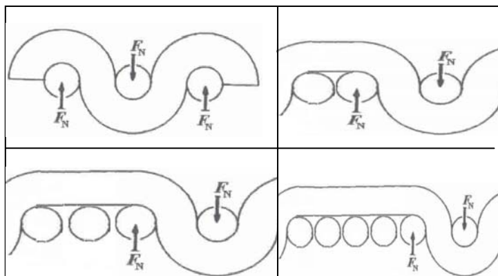
شکل ۶. شماتیک مقطع عرضی از بافت های تافته، سرزده ۲×۱، سرزده ۳×۱، سرزده ۵×۱
