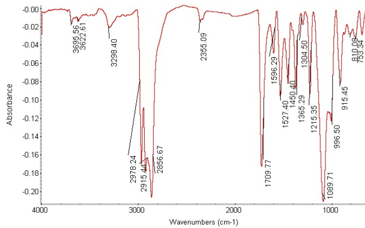
شکل ۱۸. نمودار ATR نمونه رنگ شده با راکتیو سرد عمل شده با پلازما در زمان ۱ دقیقه
