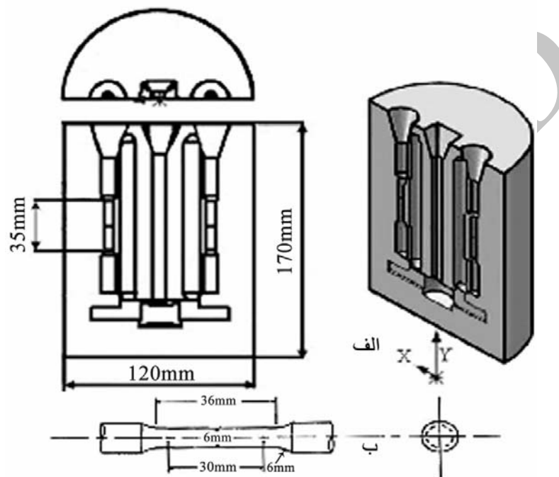
شکل ۱- الف- قالب دایمی مورد استفاده در آزمایش‌ها برای عملیات ریخته‌گری و ب- ابعاد نمونه مورد استفاده برای آزمایش کشش.
