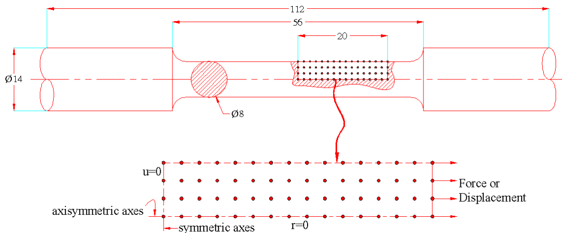
شکل ۶- ابعاد نمونه آزمون کشش و توزیع گره در حالت تقارن محوری بر حسب میلی‌متر
