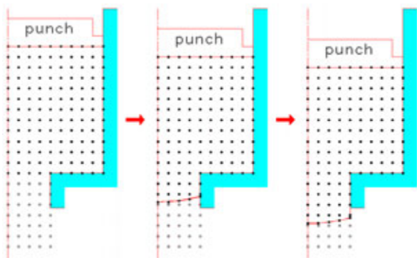
شکل ۹- چگونگی فعال‌سازی گره‌ها در مراحل گوناگون فروروی پانچ
