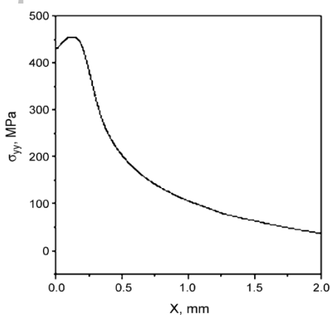
شکل ۸- توزیع بیشینه ی تنش نرمال در طول ترک برای حالت (ب).
