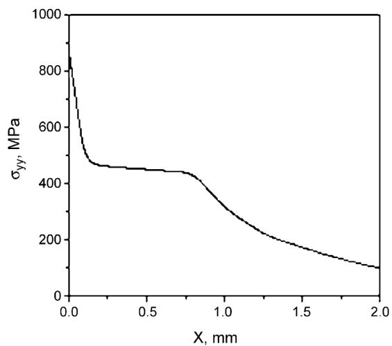
شکل ۹- توزیع بیشینه‌ی تنش نرمال در طول ترک برای حالت (ج).
