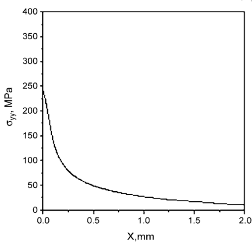
شکل ۷- توزیع بیشینه ی تنش نرمال در طول ترک برای حالت (الف).
