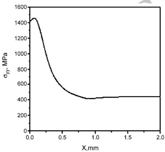
شکل ۱۰- توزیع بیشینه‌ی تنش نرمال در طول ترک برای حالت (د).
