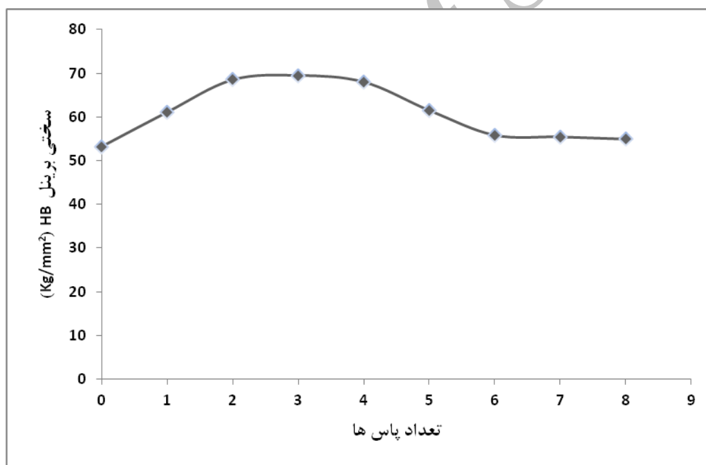
شکل 4- تغییرات سختی نمونه‌ها بر حسب تعداد مراحل اکستروژن.
