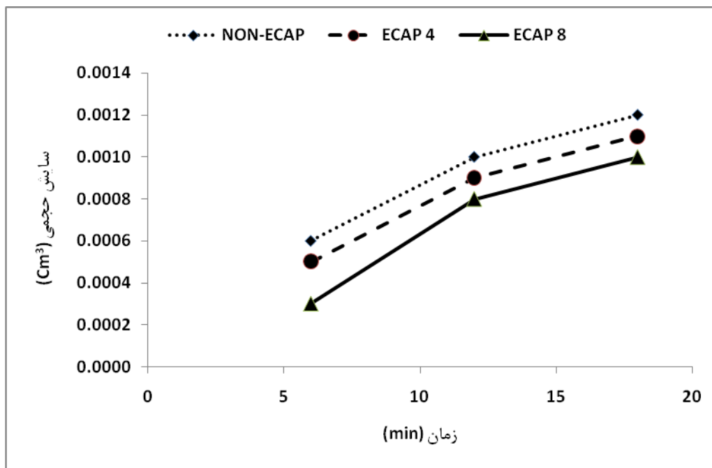
شکل 11- سایش حجمی الکترودهای مسی در شدت جریان 5 آمپر
