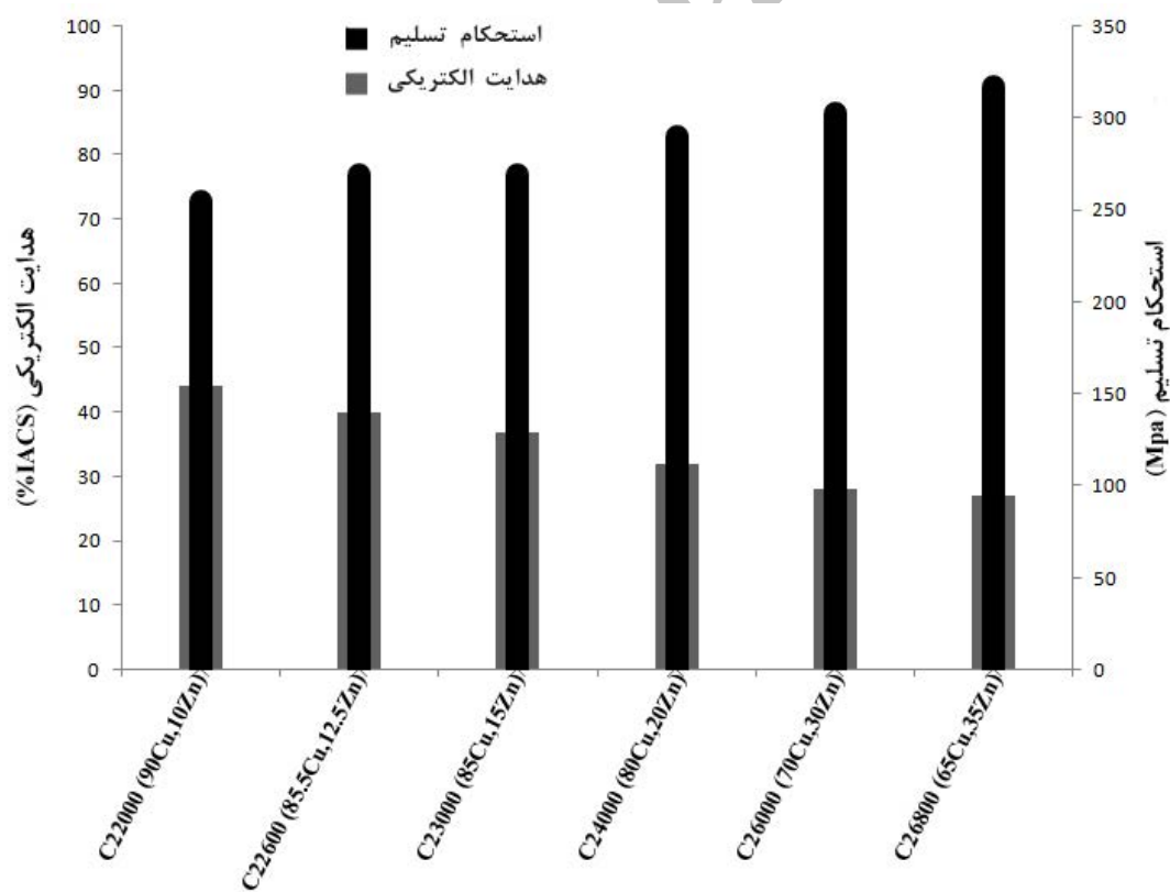
شکل 10- تغییرات هدایت الکتريکی و استحکام تسلیم مس آلیاژی (Cu-Zn) [12].
