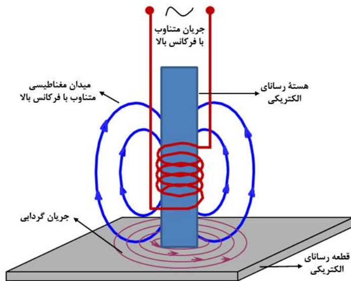
شکل 2- شماتیک روش جریان گردابی.
