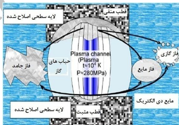
شکل 3- شرایط کاری تخلیه الکتریکی [10].
