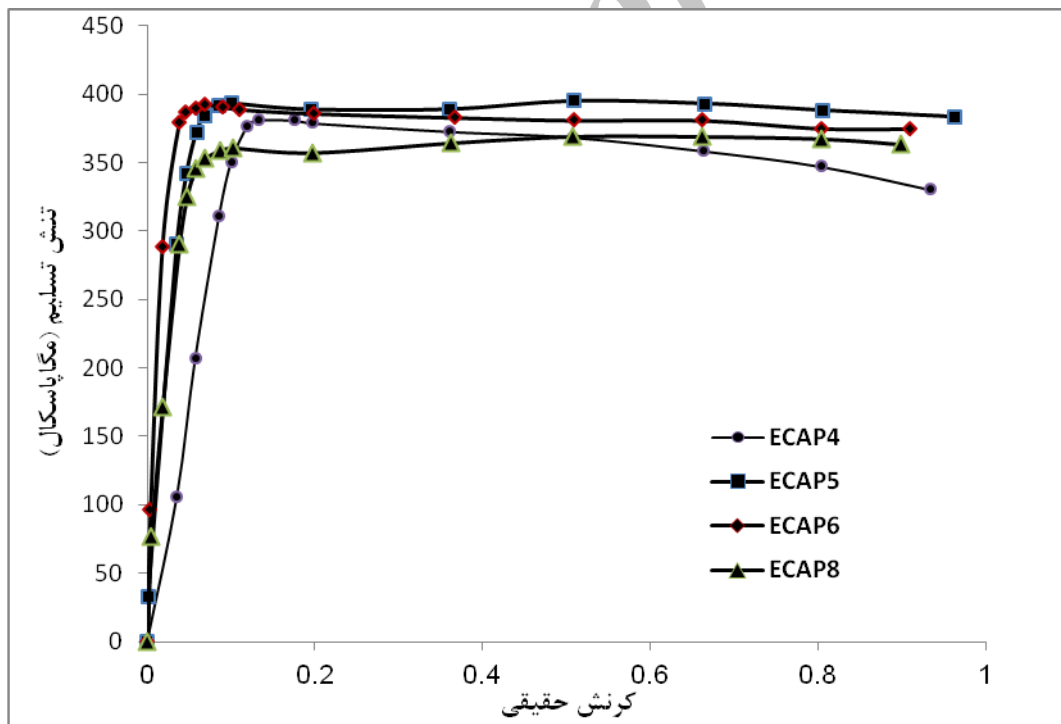
شکل 6- منحنی های تنش-کرنش فشاری مس پس از چهار تا هشت مرحله اکستروژن.
