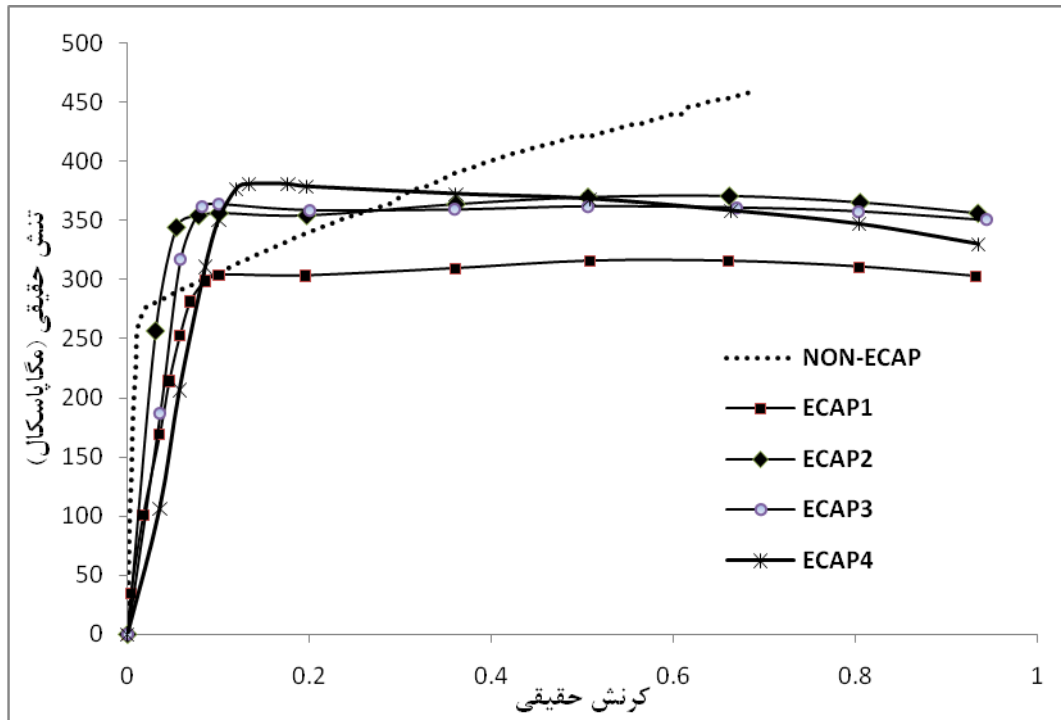
شکل 5- منحنی های تنش-کرنش فشاری مس پس از یک تا چهار مرحله اکستروژن به همراه نمونه اولیه.
