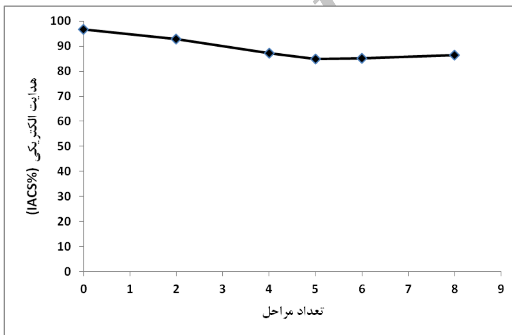
شکل 8- تغییرات هدایت الکتریکی بر حسب مراحل اکستروژن.
