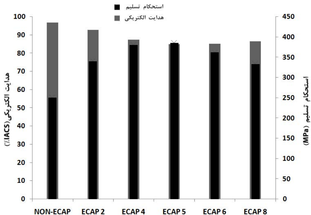
شکل 9- تغییرات هدایت الکتريکی و استحکام تسلیم مس بر حسب مراحل اکستروژن.
