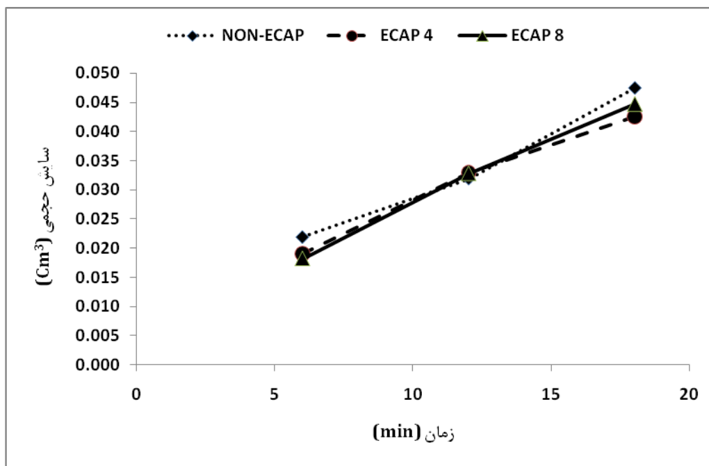
شکل 13- سایش حجمی الکترودهای مسی در شدت جریان 15 آمپر
