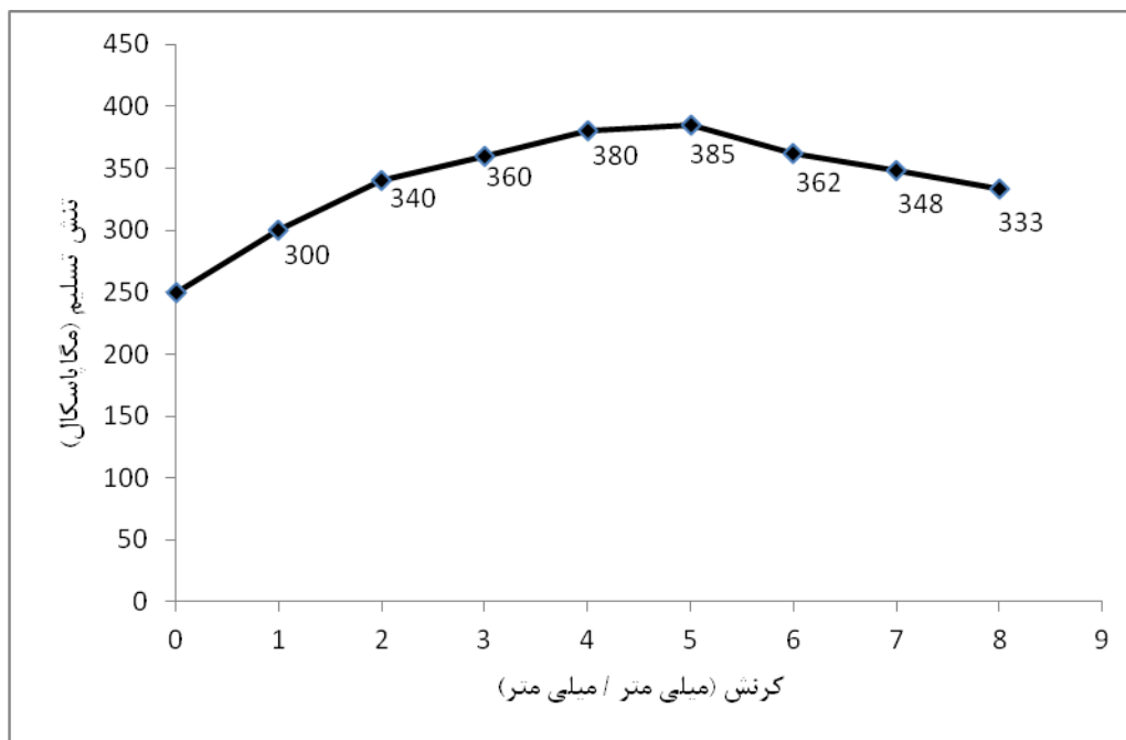
شکل 7- تغییرات تنش تسلیم مس بر حسب مراحل اکستروژن.
