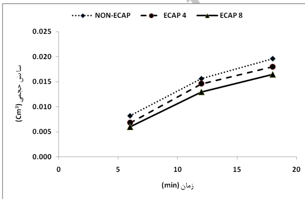
شکل 12- سایش حجمی الکترودهای مسی در شدت جریان 10 آمپر
