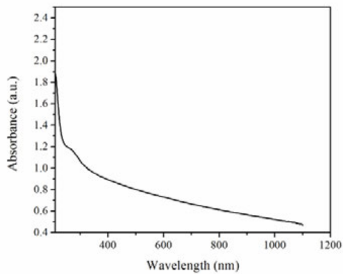
شکل 6- طیف نورسنجی (UV-visible spectroscopy) نانو ذرات اکسید قلع ساخته شده در شرایط بهینه
