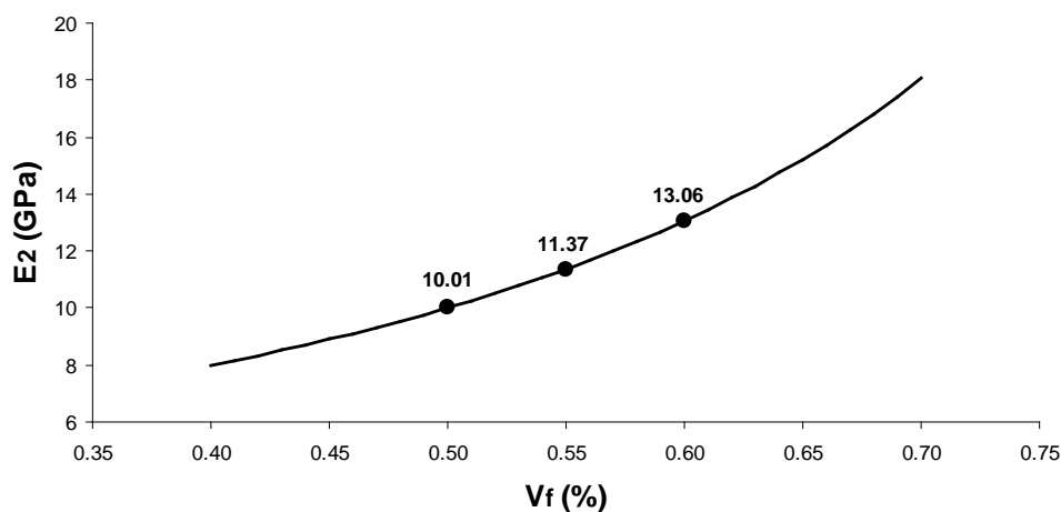
شکل 3- خروجی روابط میکرو مکانیک برای محاسبه مدول یانگ عرضی در سه کسر حجمی 50، 55 و 60 درصد از الیاف کربن.
