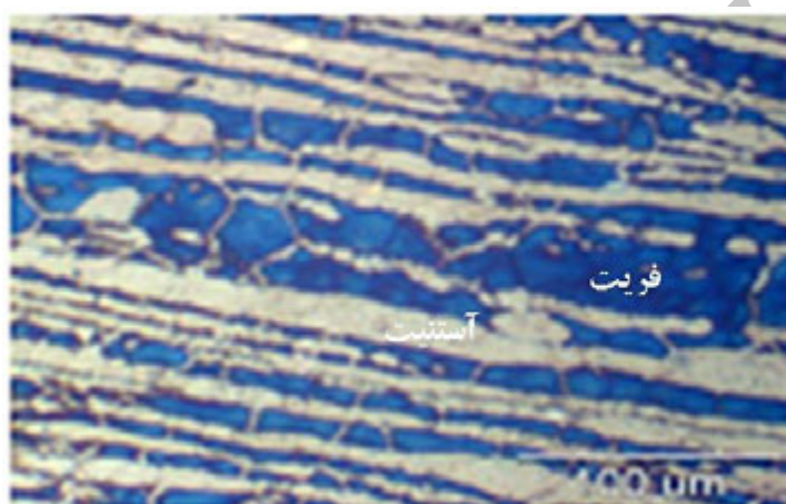
شکل 8- ریزساختار فولاد زنگ نزن سوپر دوفازی 32750.
