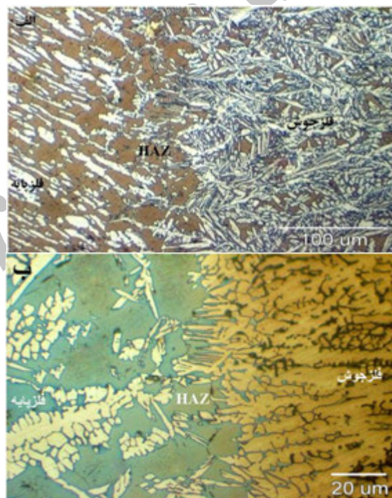
شکل 8- (الف) فصل مشترک بین فلز پایه آستنیتی 32750 و فلز جوش 25104L مربوط به پاس نخست. (ب) فصل مشترک بین فلز پایه آستنیتی 32750 و فلز جوش 309LMo مربوط به پاس نخست.
