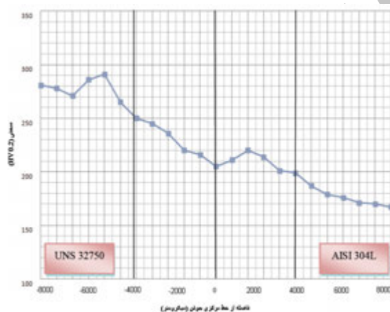
شکل 88- پروفیل سختی مقطع جوش نامشابه فولاد زنگ نزن آستنیتی 304L به فولاد زنگ نزن سوپر دوفازی 32750 با استفاده از فلز پرکننده 309LMo.
