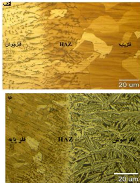
شکل 7- (الف) فصل مشترک بین فلز پایه آستنیتی 304L و فلز جوش 309LMo مربوط به پاس نخست. (ب) فصل مشترک بین فلز پایه آستنیتی 304L و فلز جوش 25104L مربوط به پاس نخست.
