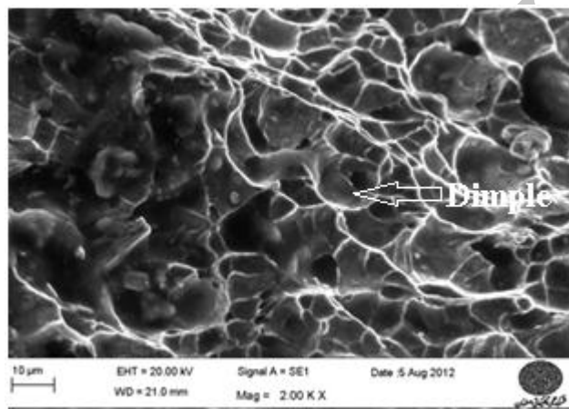
شکل 81 - شکست نگاری فلز جوش ER25104L با بزرگنمایی 2111 برابر.
