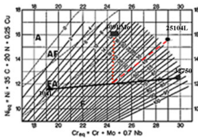
شکل 6- نمودار WRC-1992 برای فولادهای زنگ نزن دوقازی [8].
