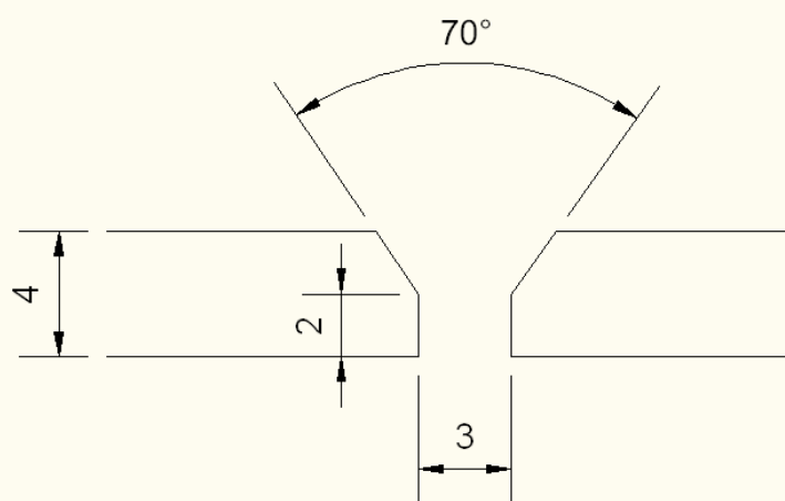
شکل 8- طرح اتصال لوله ها.
