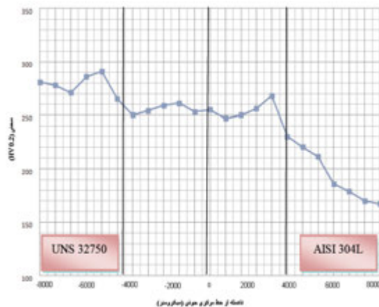
شکل 82- پروفیل سختی مقطع جوش نامشابه فولاد زنگ نزن آستنیتی 304L به فولاد زنگ نزن سوپر دوفازی 32750 با استفاده از فلز پرکننده 25104L.
