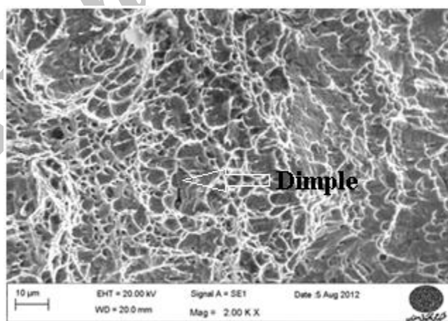
شکل 88 - شکست نگاری فلز جوش ER309LMo با بزرگنمایی 2111 برابر.
