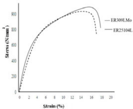
شکل 9- نمودار تنش بر حسب کرنش مربوط به اتصالات.
