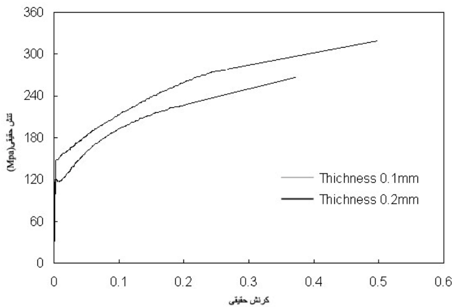
شکل ۷- مقایسه نمودارهای تنش- کرنش حقیقی در ضخامت‌های ۰/۲ و ۰/۱ میلیمتر
