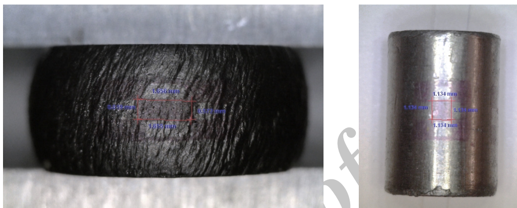
شکل ۲- نمونه‌ها پس از انجام آزمایش اریکسون
