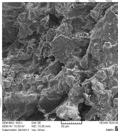
شکل ۱۲- تصویر میکروسکپ الکترونی از سطح شکست کامپوزیت تهیه شده با درصد‌های مناسب و بهینه از مواد اولیه مصرفی (۳۰ درصد وزنی گرافیت، ۴۲ درصد وزنی کاربید سیلیسیم، ۱۹/۶ درصد وزنی کائولن زلیتیز و ۸/۴ درصد وزنی تالک لوزاناک).
