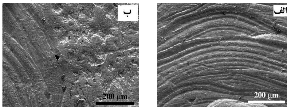
شکل ۴- تصویر میکروسکوپ الکترونی روبشی از محل جوش لیزری تیتانیوم (الف) خط جوش (ب) منطقه متاثر از حرارت
