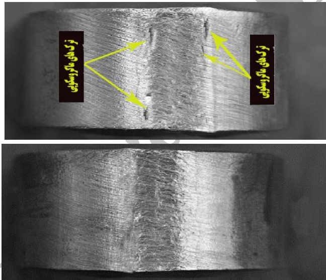
شکل ۹- تصاویر میکروسکوپی از نمونه‌های تست خمش الف) جوشکاری GTAW ب) جوشکاری لیزر
