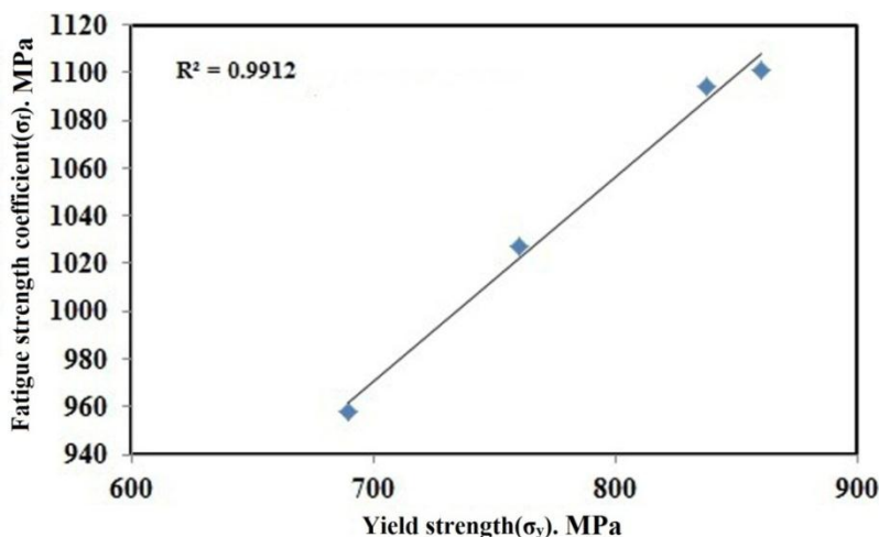
شکل ۷-۱ ارتباط بین ضریب استحکام خستگی و استحکام تسلیم.
