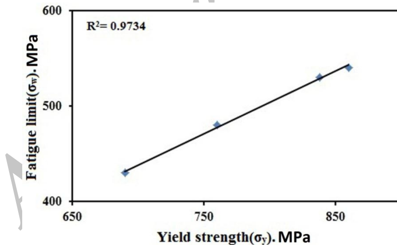
شکل ۶- ارتباط بین حد خستگی و استحکام تسلیم.
