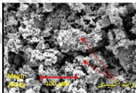
شکل ۱۰- تصویر میکروسکوپ الکترونی از ذرات بدست آمده از سایش نمونه ۱.
