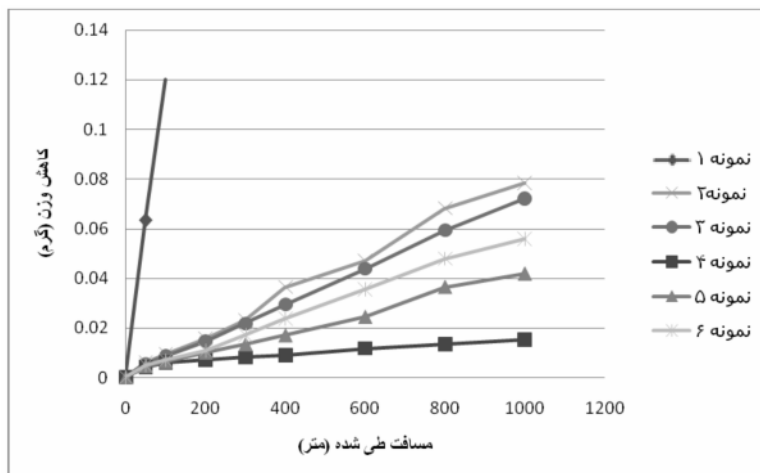
شکل ۱۱- نمودار کاهش وزن بر حسب مسافت طی شده برای نمونه‌های آزمون سایش.
