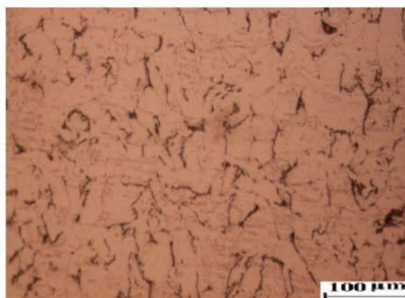
شکل ۱- ریزساختار فولاد ASTM A106-Gr.B
