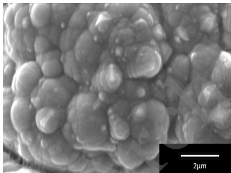
شکل ۴- تصویر بزرگ شده ساختار گل کلمی شکل پرمالوی (۸ ساعت آیکاری در دمای ۲۵ درجه سانتی‌گراد در حضور ۱g/L ساخارین و همزن مکانیکی)
