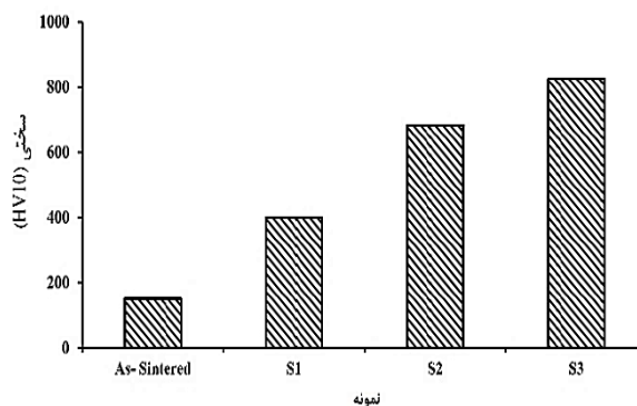
شکل ۸- نتایج ماکروسختی نمونه‌های ذوب سطحی شده
