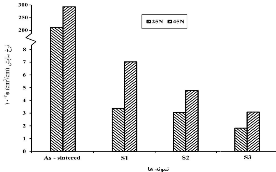
شکل ۹- نرخ متوسط ساییش فولاد پایه و نمونه های ذوب سطحی شده در نیروهای اعمالی ۲۵ و ۴۵ نیوتن
