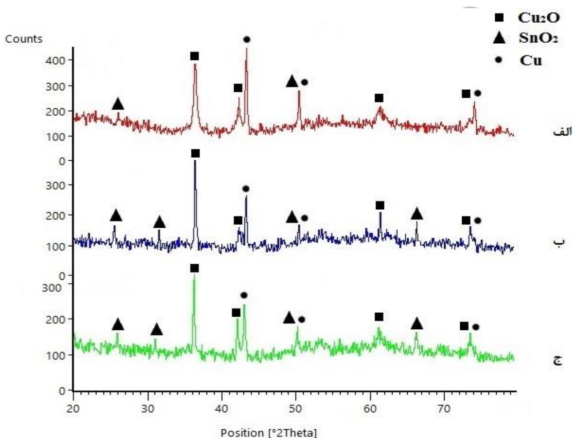
شکل ۱- طیف پراش اشعه ایکس نانو ذرات اکسید مس - قلع سنتز شده (الف) جریان ۵۰۰، (ب) جریان ۲۵۰
