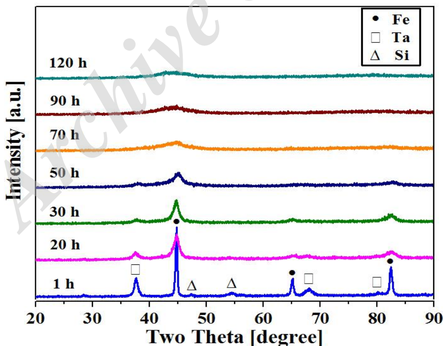
شکل ۱- الگوی XRD آلیاژ Fe_{75}Ta_5Si_{10}C_{10} در زمان‌های مختلف آسیاکاری پس از افزودن PCA
