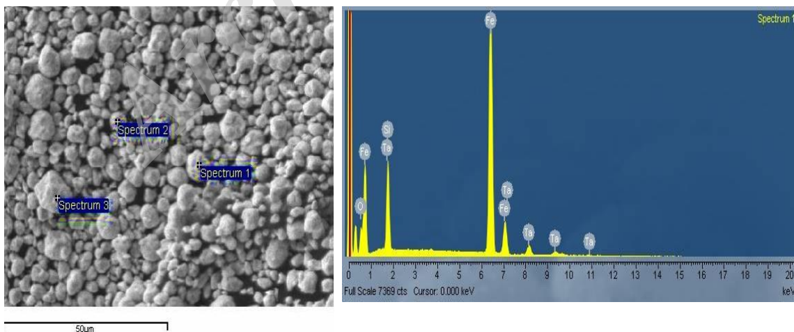
شکل ۸- آنالیز EDS و تصویر SEM مربوطه پودر آلیاژ تولید شده با PCA پس از ۱۲۰ ساعت فرایند آلیاژسازی مکانیکی
