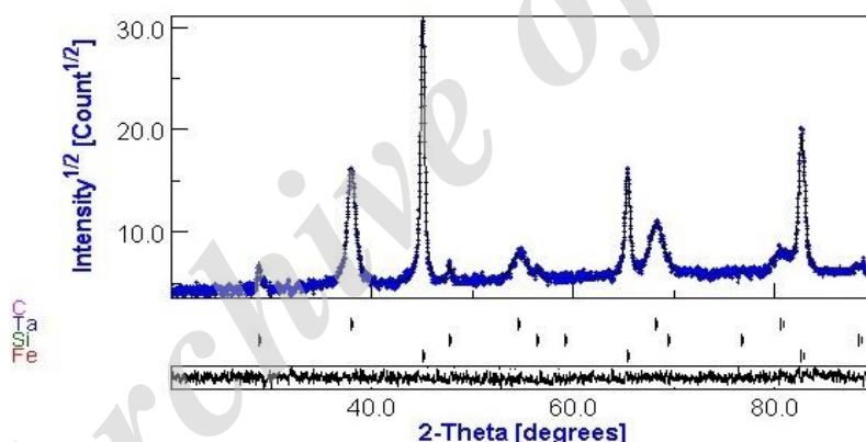
شکل ۲- الگوی XRD نمونه ۱ ساعت آسیاکاری و برازش شده توسط نرم افزار MAUD با مقادیر R_{wp}=10/52 و R_{exp}=9/93 که به ترتیب فاکتور باقیمانده وزن شده و مورد انتظار می‌باشند. اختلاف بین الگوی آزمایشگاهی و آنالیز شده زیر رسم شده است
