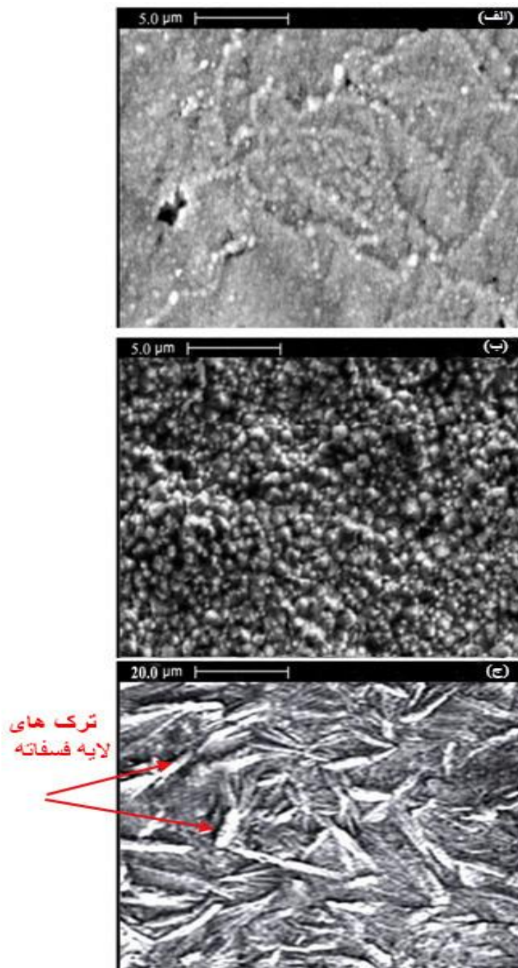
شکل ۳-الف) تصویر SEM از ساختار پوشش به دست آمده از حمام (۱)، ب) تصویر SEM از ساختار پوشش به دست آمده از حمام (۲)، ج) تصویر SEM از پوشش فسفات
