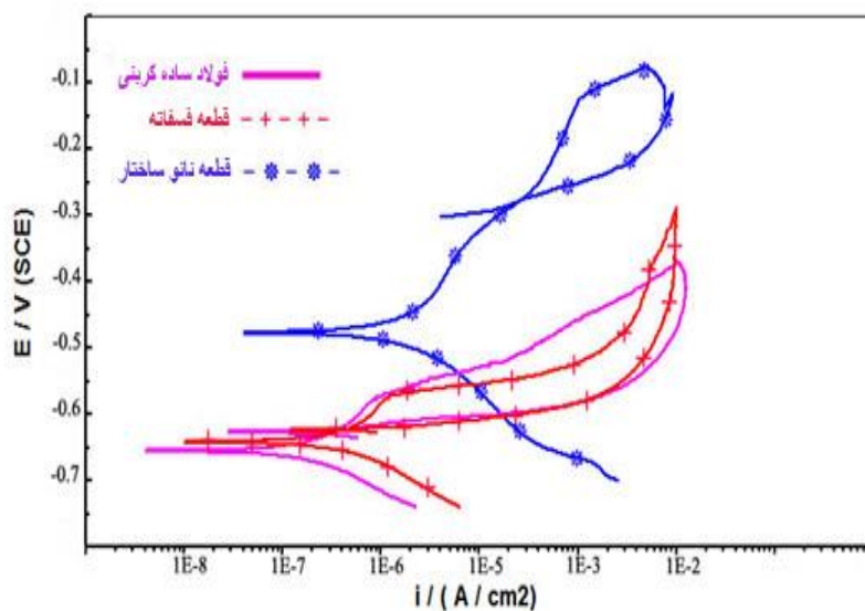
شکل ۵- نمودار پلاریزاسیون سیکی برای نمونه‌های با دو نوع پرایمر استفاده شده
