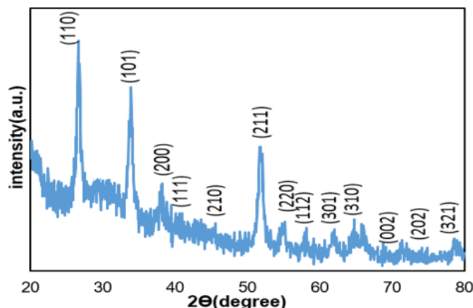
شکل ۵- الگوی XRD مربوط به نمونه Zn doped SnO 2 سنتز شده در دمای ۲۰۰ C° بعد از کلسینه شدن در دمای ۶۰۰ C° برای مدت زمان ۲ ساعت
