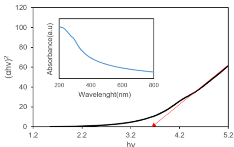
شکل ۷- نمودار شکاف انرژی برای نمونه Zn-doped SnO 2 سنتز شده در دمای ۲۰۰ C° بعد از کلسینه شدن در دمای C° ۶۰۰ برای مدت زمان ۲ ساعت
