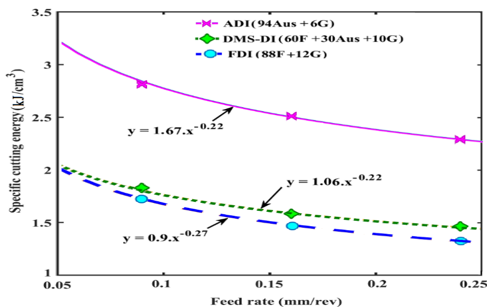
شکل ۸- تغییرات انرژی مخصوص برش نمونه‌های FDI، DMS و ADI با نرخ پیشروی
