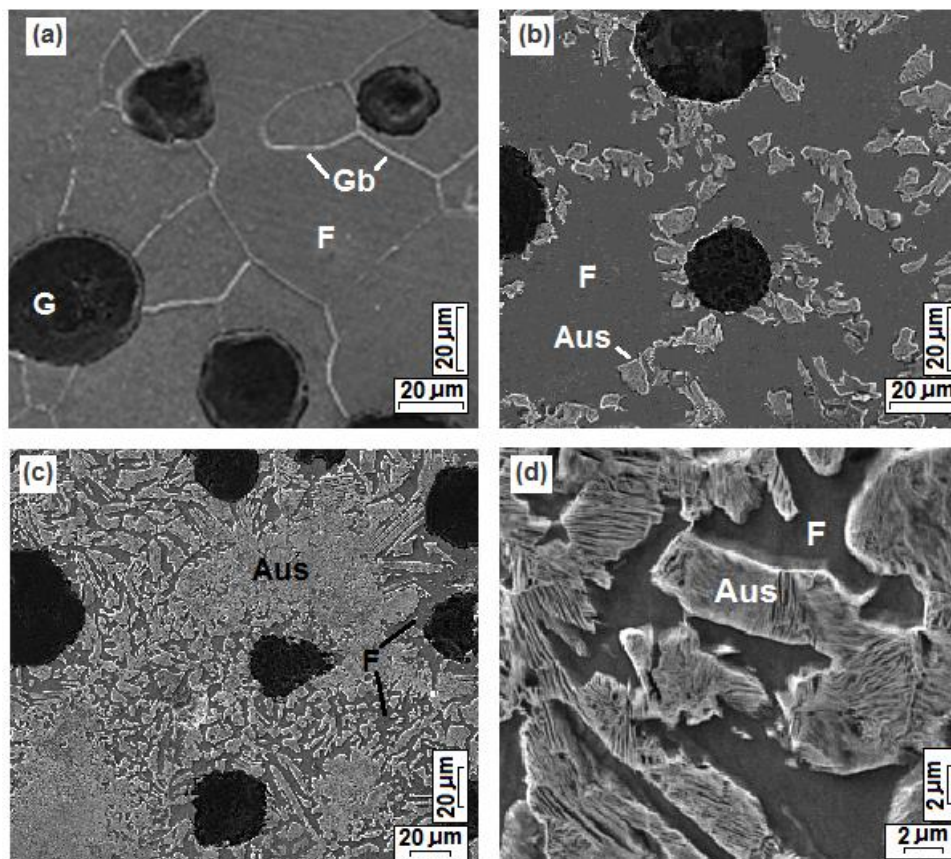
شکل ۳- تصاویر میکروسکوپی الکترونی روبشی (a) نمونه ریختگی، (b) و (c) به ترتیب نمونه‌های آستنیت‌زدگی شده به مدت ۱۲ min و ۲۰ min و سپس آستمپر شده (d) فازهای فریت (تیره رنگ) و آسفریت در بزرگنمایی بالا
