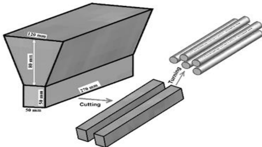
شکل ۱- نمایش قالب Y بلوک مورد استفاده و ابعاد آن
