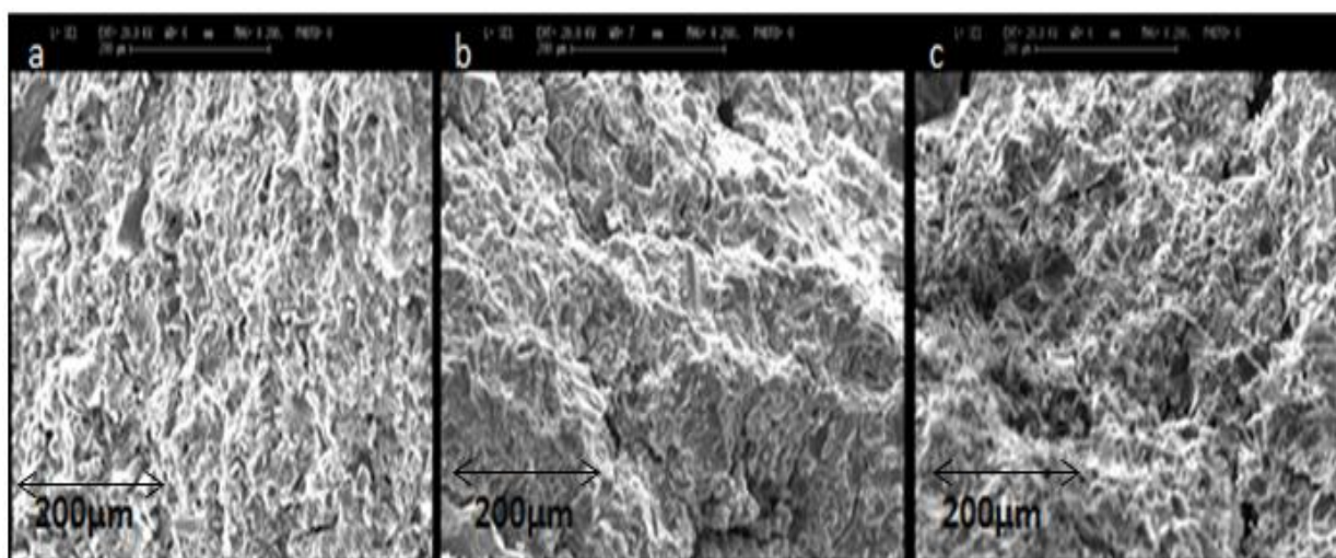
شکل ۱۲- تصاویر SEM، (a) نمونه شاهد (b) نمونه حاوی ۵ درصد اکسید بور (c) نمونه حاوی ۵ درصد کاربید بور
