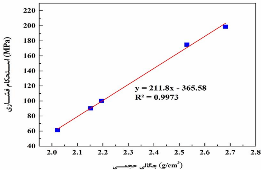
شکل ۸- نمودار تغییرات استحکام فشاری بر حسب چگالی حجمی آن‌ها
