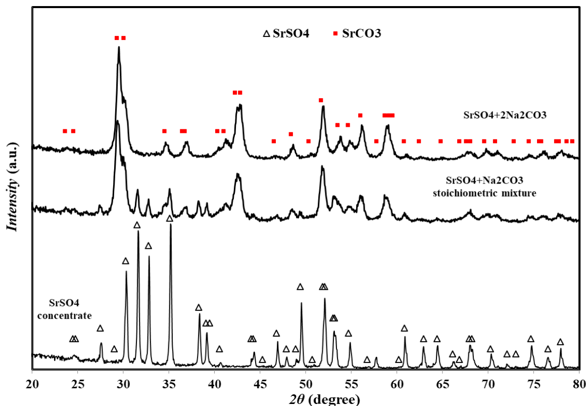
شکل ۲- نتایج آنالیز اشعه ایکس کنسانتره سلسیتیت و باقی مانده جامد مخلوط‌های آسیاکاری شده سلسیتیت-کربنات سدیم پس از انحلال در آب. نمونه کنسانتره سلسیتیت با خلوص بیش از ۹۸٪ (الگوی پایین)، مخلوط \text{SrSO}_4+\text{Na}_2\text{CO}_3 با نسبت استوکیومتری و مخلوط \text{SrSO}_4+2\text{Na}_2\text{CO}_3 با نسبت دو برابر مولی کربنات سدیم در مخلوط (الگوی بالا)
