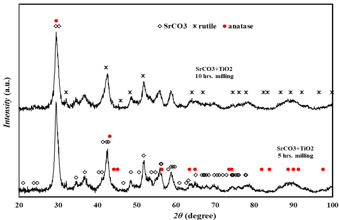
شکل ۳- نتایج الگوهای پراش اشعه ایکس مخلوط های کربنات استرانسیم-دی اکسید تیتانیم پس از پنج و ده ساعت آسیاکاری مکانیکی
