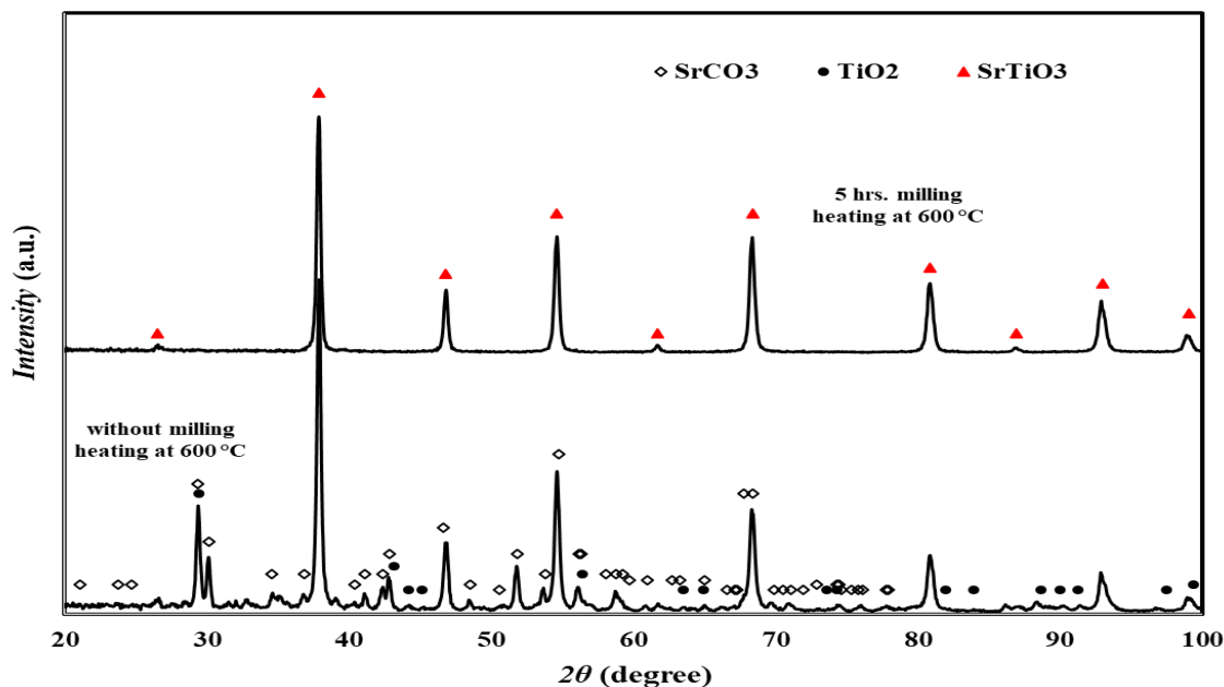
شکل ۵- الگوی پراش اشعه ایکس باقی مانده جامد مخلوط بدون آسیاکاری و مخلوط پنج ساعت آسیاکاری پس از گرمایش همدمای به مدت یک ساعت دردمای ۶۰۰ درجه سانتیگراد
