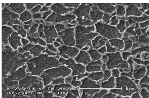
شکل ۹- تصویر میکروسکوپ الکترونی روبشی از ریزساختار فولاد ساده کربنی بعد از تغییر شکل پلاستیک شدید در دمای پیشگرم ۹۳۰ درجه سانتیگراد
