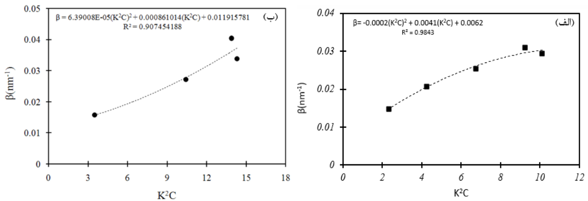
شکل ۷ - تغییرات عرض انتگرالی پیک‌های پراش پرتو ایکس به صورت تابعی از K^2C برای نمونه‌های Ex-ECAP شده: الف) آلایژ آلومینیم ۷.۷۵، ب) فولاد ساده کربنی فریتی
