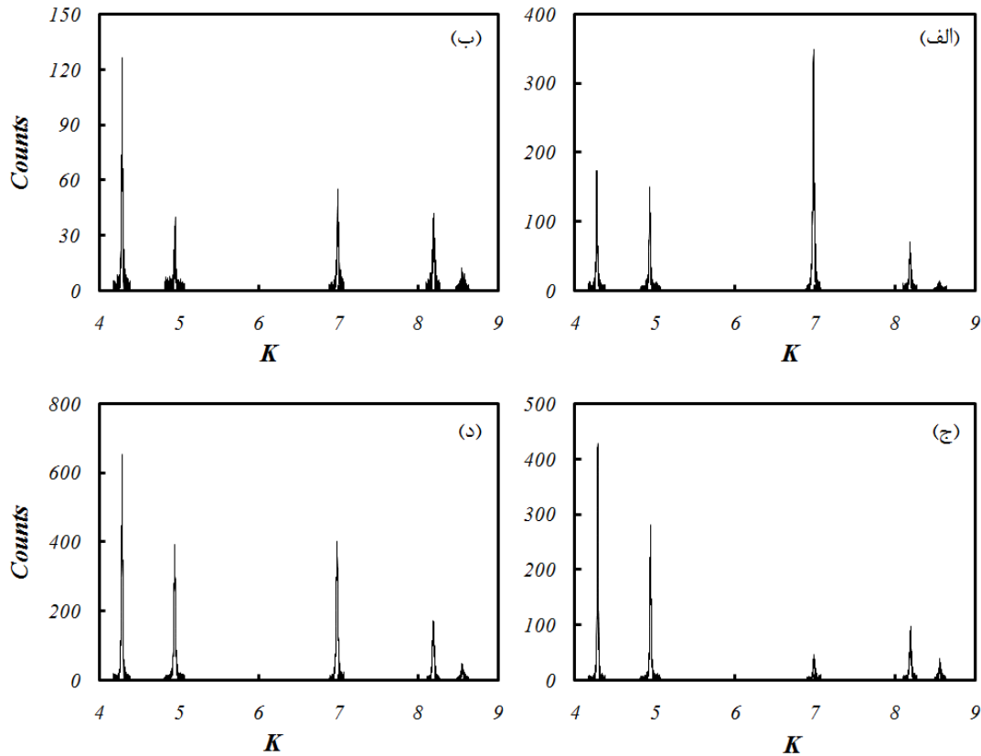
شکل ۶- الگوی پراش پرتوی ایکس نمونه آلومینیم ۷.۷۵ بعد از Ex-ECAP در دمای محیط در سه صفحه مختلف: الف) X (ب) Y، ج) Z و د) الگوی پراش مجموع سه صفحه
