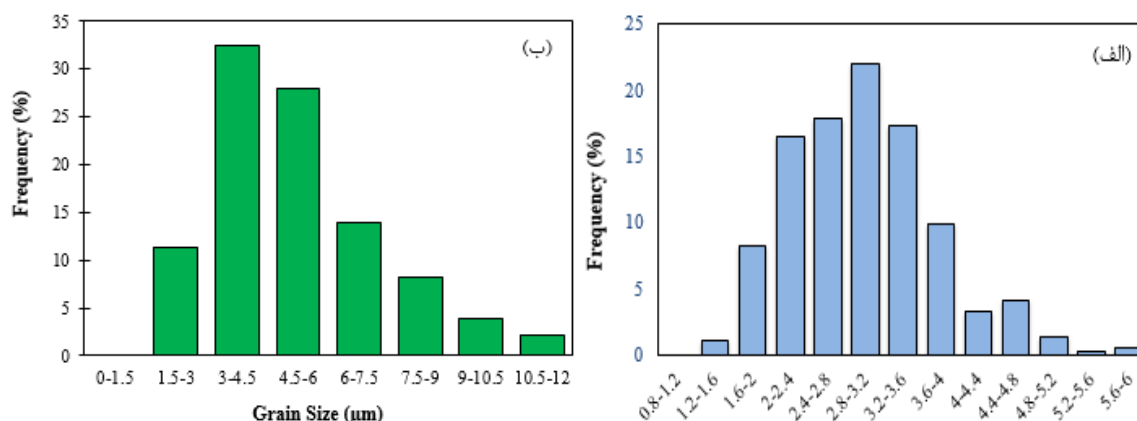
شکل ۱۰- توزیع اندازه دانه در ساختار حاصل از تغییر شکل دما بالا به روش Ex-ECAP: الف) فولاد ساده کربنی، ب) آلیاژ آلومینیوم ۷۰۷۵
