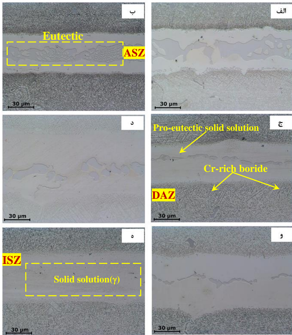
شکل ۵- ریزساختار نواحی مختلف اتصال GTD111/BNi-3/GTD111 در دمای ۱۱۶۰°C زمان‌های: الف) ۵، ب) ۱۵، ج) ۳۰، د) ۶۰، و) ۷۵ و ه) ۹۰ دقیقه
