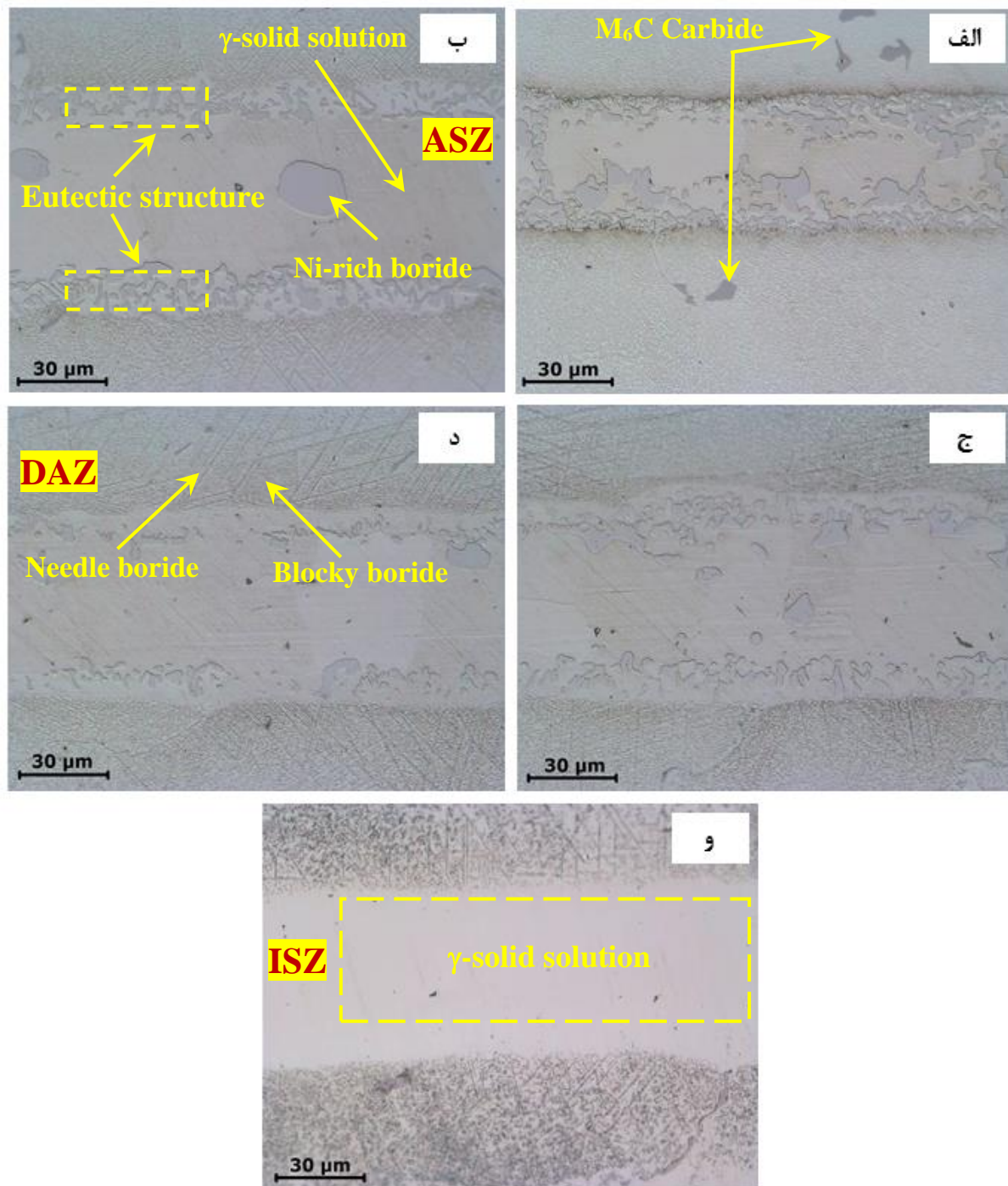
شکل ۳- ریزساختار نواحی مختلف اتصال GTD111/BNi-3/GTD111 در دمای ۱۰۸۰°C زمان‌های: الف) ۱۵، ب) ۱۵۰ و ج) ۱۶۵، د) ۱۸۰ و ه) ۱۹۵ دقیقه
