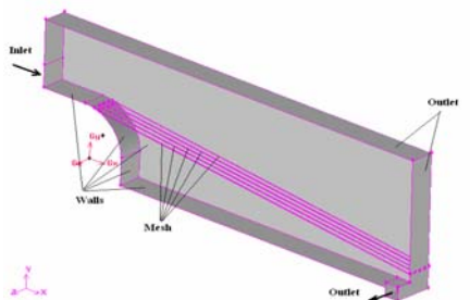
شکل ۷- آشغالگیر سه بعدی همراه با شبکه ی آشغالگیر و شرایط مرزی.
