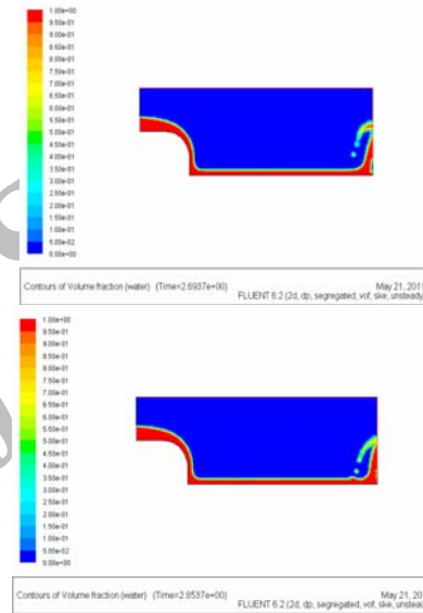
شکل ۱۰- نحوه ی پر شدن آشغالگیر و ایجاد جریان گردابی پس از برخورد آب با دیواره، در آشغالگیر بعدی و سه بعدی.
