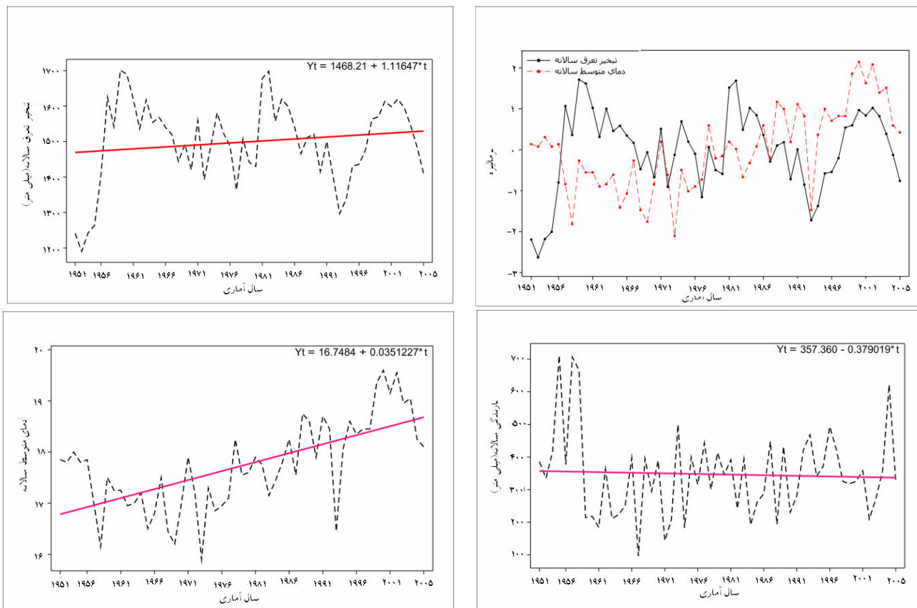
شکل ۲- تغییرات تبخیر- تدریج گیاه مرجع، بارندگی و میانگین دمای سالانه در ایستگاه سینوپتیک شیراز.
