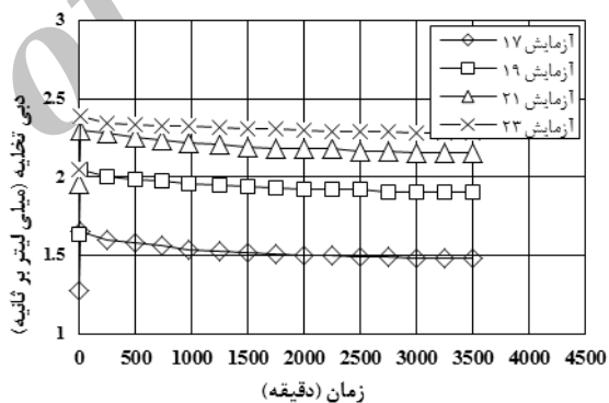
شکل ۱۲: بدهی تخلیه در سامانه‌ی صافی با ژئوتکستایل G_1 آزمایش شده با خاک S_1 و صفحات سوراخدار.
