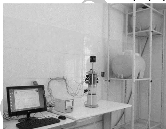
شکل ۶: مجموعه‌ی دستگاههای آزمایش نفوذپذیری.
