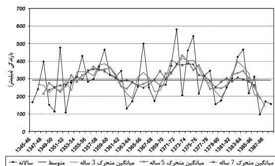
شکل 3. نمودار میانگین متحرک بارندگی ایستگاه فسا
