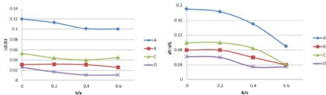
شکل 8- متوسط بیشترین اختلاف عمق آب به عمق آب در ابتدای سرریز و میانگین نرخ افزایش سرعت در سرریز های گروههای A، B، C و D در سرریز های ساده (با نسبت شعاع کوچک به شعاع بزرگ برابر صفر)، و سرریز های نیمه بیضوی با نسبت شعاع کوچک به شعاع بزرگ (b/a) برابر 0/2، 0/4 و 0/6.
