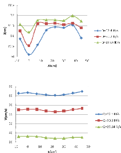
شکل 4- تراز سطح آب و نیمرخ سرعت در یک نمونه سرریز.
