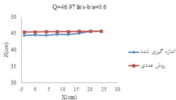
شکل 10- نیمرخ‌های به‌دست آمده از حل عددی معادله پویایی و مقادیر اندازه گیری شده در یک نمونه‌ی سرریز گروه B.
