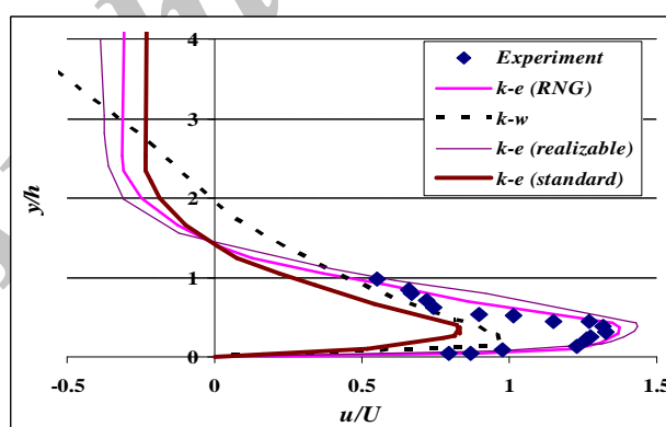
شکل 5- مقایسه‌ی نیمرخ قائم سرعت موضعی آزمایش SAL26 در الف) وضعیت فوق بحرانی پیش از پرش و در ب) وضعیت زیربحرانی بعد از پرش چگال.
