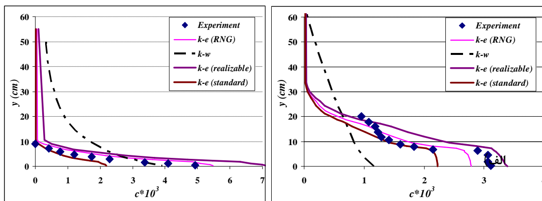
شکل 4- مقایسه‌ی نیمرخ قائم غلظت موضعی آزمایش SAL29 در موقعیت الف) و ب) 9 متری از دریچه‌ی کشویی.
