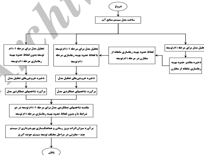
شکل ۱: نمودار گردش‌ی ۱ تعیین میزان اثرات به‌روزرسانی و هماهنگ‌سازی بهره‌برداری از سامانه‌ی آبی حوضه‌ی آبخیز در مراحل مختلف توسعه.
