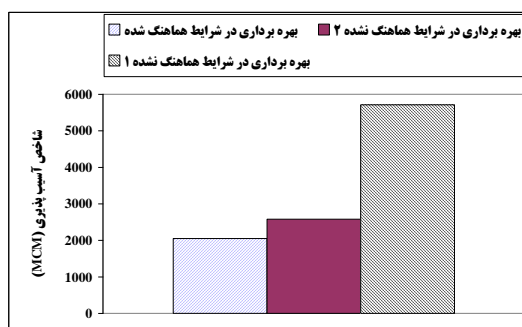
شکل ۹: شاخص آسب‌پذیری بهره‌برداری از سامانه‌ی آبی حوضه‌ی آبخیز کرخه در شرایط مختلف هماهنگ‌شده و هماهنگ نشده.
