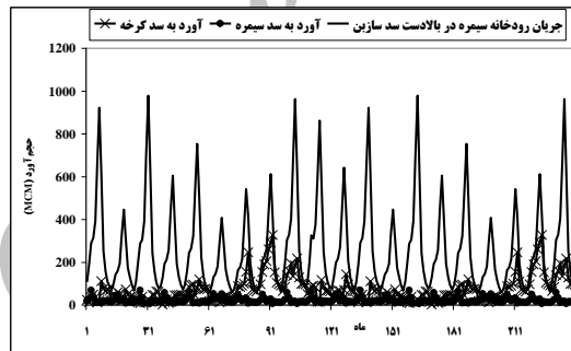
شکل ۷: آورده‌های ۲۰ ساله در سامانه‌ی آبی حوضه‌ی آبخیز کرخه.
