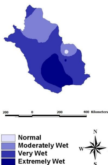
شکل ۱۱- پهنه‌بندی خشکسالی گندم در استان فارس با دوره‌ی بازگشت ۵۰ سال (بر اساس طبقه‌بندی شاخص RDI_S ).
