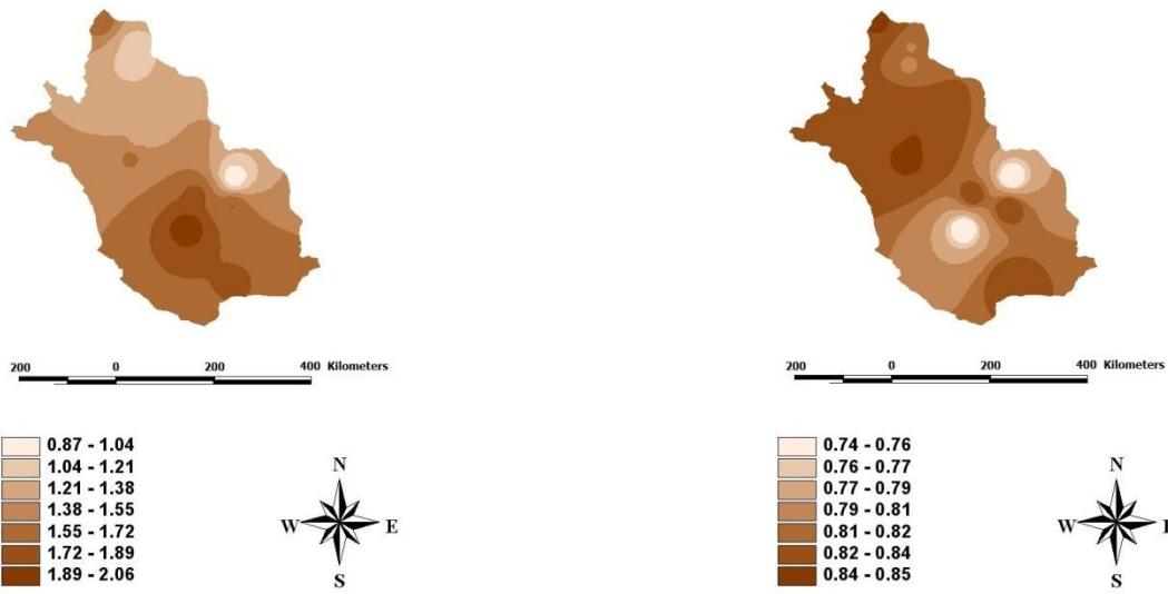
شکل ۵- پهنه‌بندی خشکسالی گندم در استان فارس با دوره‌ی بازگشت ۵ سال (بر اساس شاخص RDI_S ).
