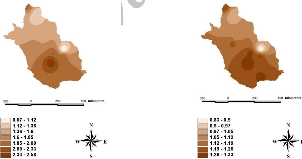
شکل ۶- پهنه‌بندی خشکسالی گندم در استان فارس با دوره‌ی بازگشت ۱۰ سال (بر اساس شاخص RDI_S ).
