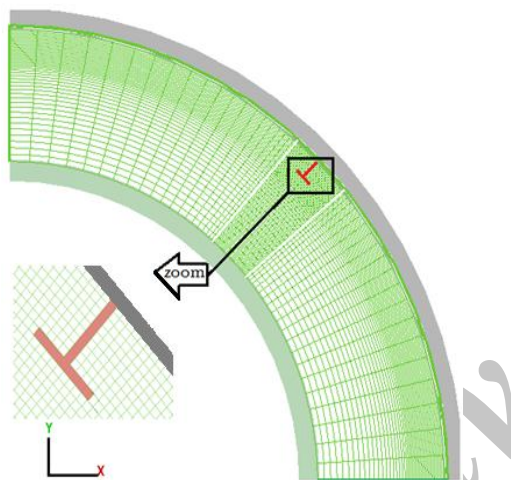
شکل ۲- طرح‌واره‌ای از شبکه‌بندی تولید شده
