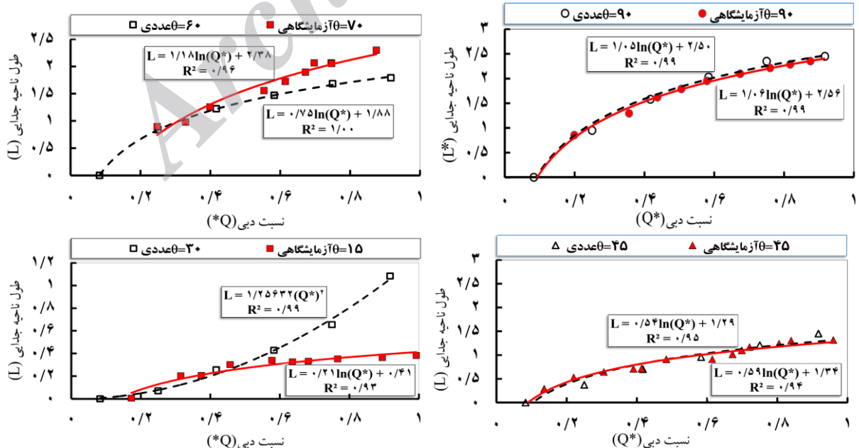
شکل ۸- تغییرات طول ناحیه‌ی جدایی جریان تحت تأثیر نسبت بده در سطح آب
