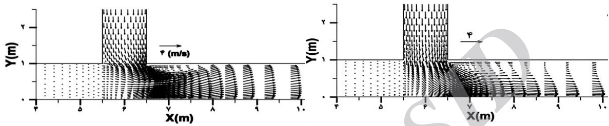
شکل ۷- بردارهای سرعت و خطوط جریان در نتایج عددی در نهر متقاطع (تحقق حاضر) الف) نزدیک سطح ( Z^*=0/95 ) ب) نزدیک کف ( Z^*=0/05 ) ج) نزدیک سطح ( Z^*=0/95 ) د) نزدیک کف ( Z^*=0/05 )
