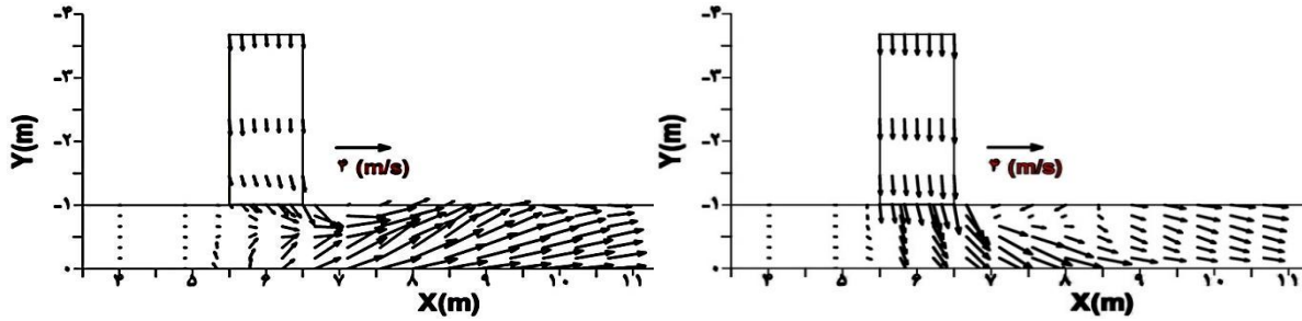
شکل ۶- بردارهای سرعت در نتایج آزمایشگاهی (Weber et al., 2001) نهر متقاطع الف) نزدیک سطح ( Z^*=0/95 ) ب) نزدیک کف ( Z^*=0/05 )
