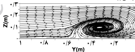
شکل ۵- جریان چرخش در محل تقاطع نه‌ها
