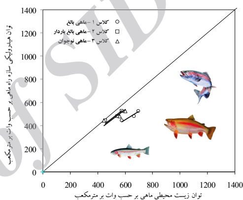
شکل ۳. مقایسه توان هیدرولیکی سازه راه ماهی با توان زیست محیطی ماهی بر حسب وات بر مترمکعب
