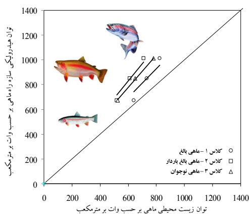
شکل ۴. مقایسه توان هیدرولیکی سازه راه ماهی با توان زیست محیطی ماهی بر حسب وات بر مترمکعب
