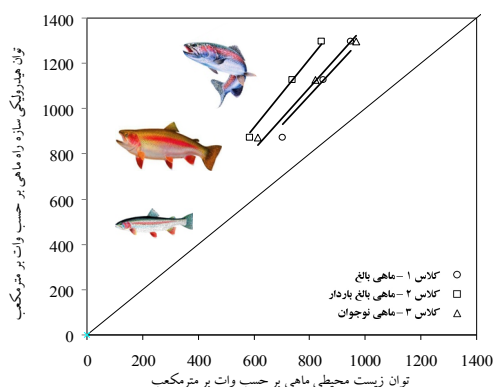
شکل ۲. مقایسه توان هیدرولیکی راه ماهی با توان زیست محیطی در بخش خروجی تحت زاویای مختلف قاب
